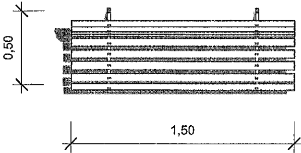
2 Planta baixa 1 : 25
