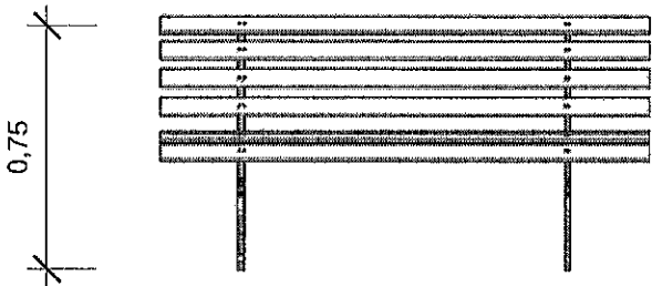
3 Elevação frontal 1 : 25
